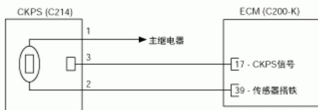
[电路图]
